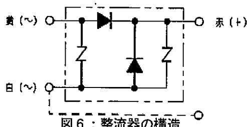
図6：整流器の構造
