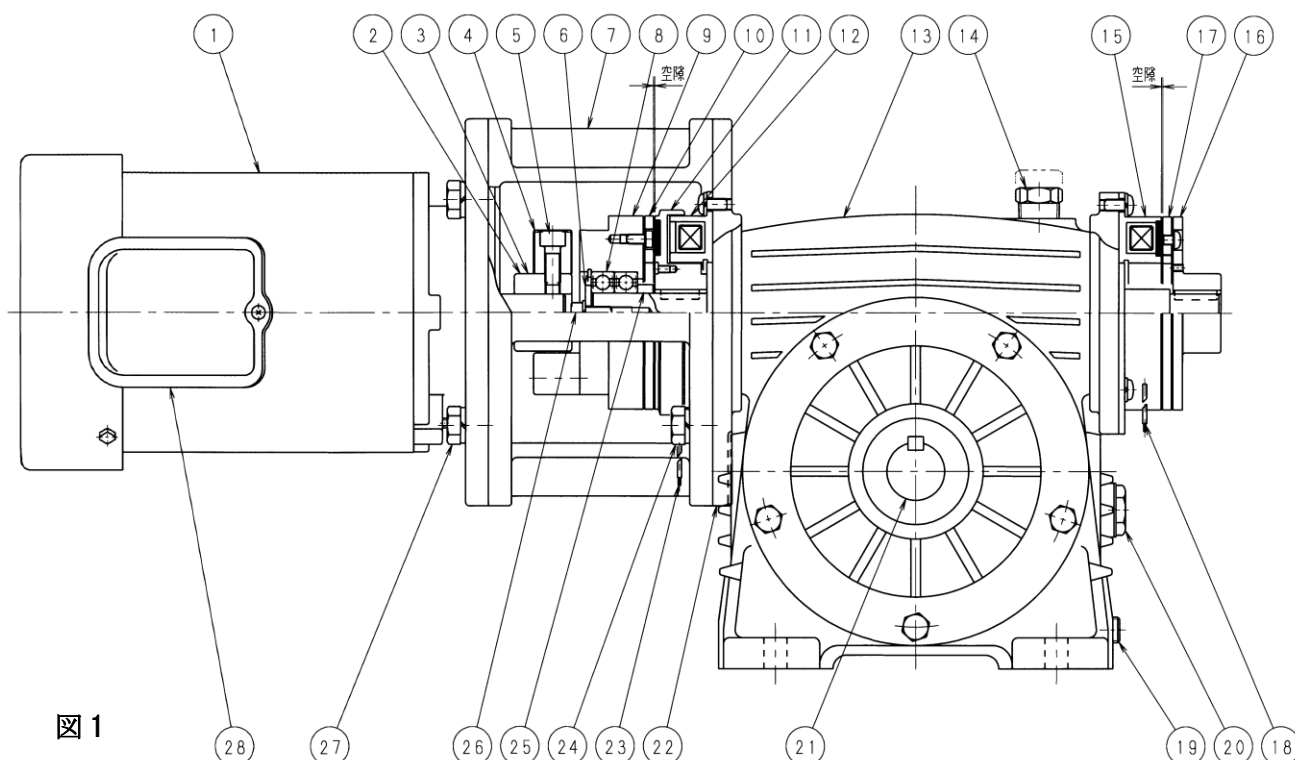
4-1 構造図
