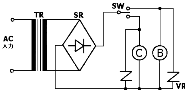
図2 結線図
