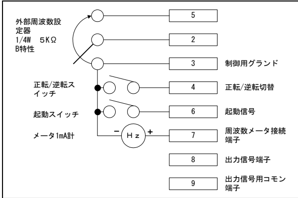
VFD-□□Aの接続例
